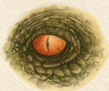
Глаз Радужка и вертикальный зрачок
