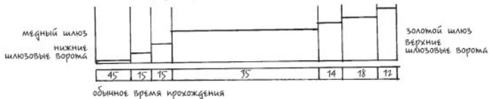
Профиль шлюзов Лукуры согласно королевскому указу средний уровень в период летней межени
